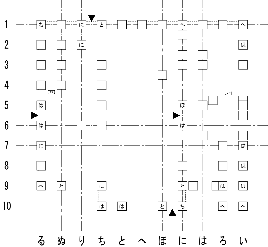
1階柱壁伏図
