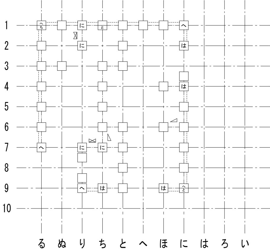
2階柱壁伏図
